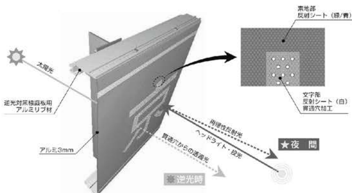
■ 逆光対策標識板の構成
